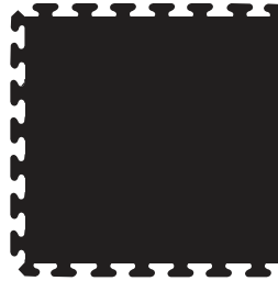
Center tile
