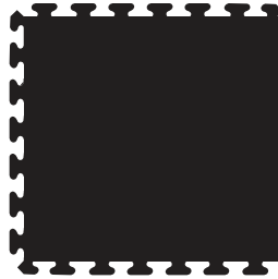
Border tile
